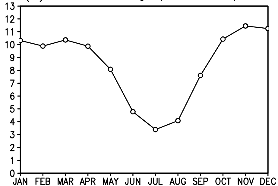
(d) Mean SAT change (Arctic Ocean)
