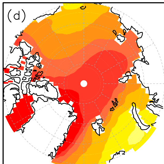
LW_water vapour
