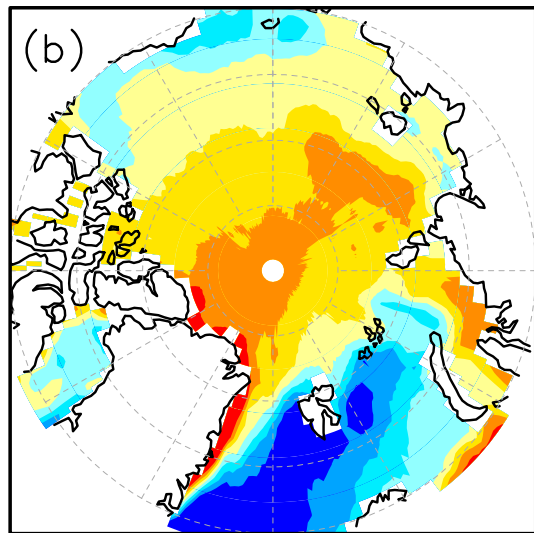
LW_cloud
