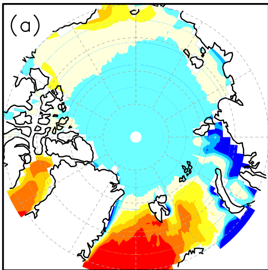
SW_cloud
