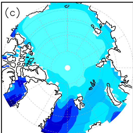
SW_water vapour
