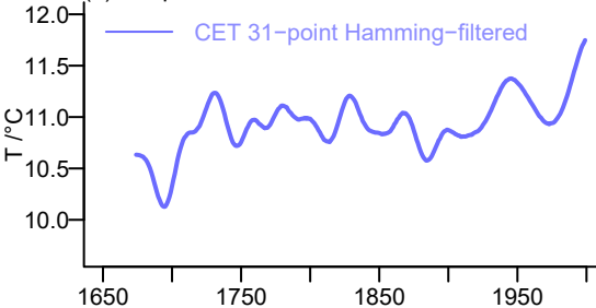
(d) Temperature
